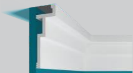
P101 13 x 4,5 x 200 см
