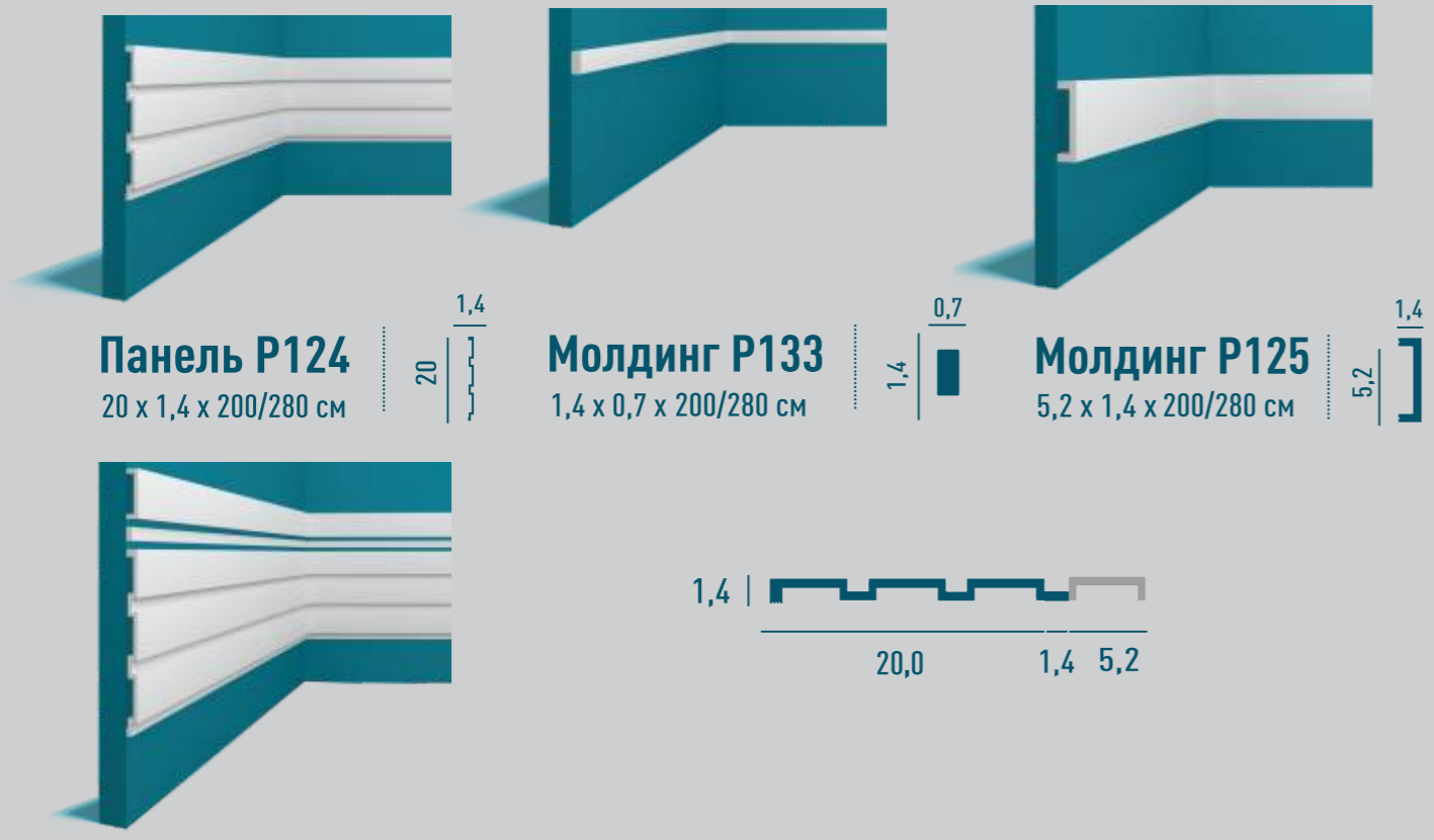
Панель P124 + Молдинг P133 + Молдинг P125
