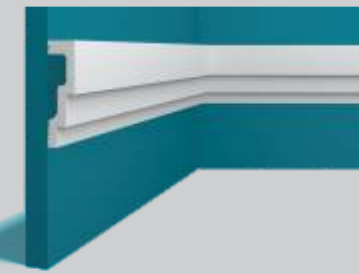
P106 7 x 2 x 200 cm
